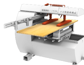
Stabilno držanje panela i preciznost bušenja
